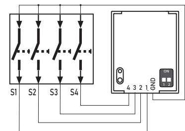
Anschluss Taster
